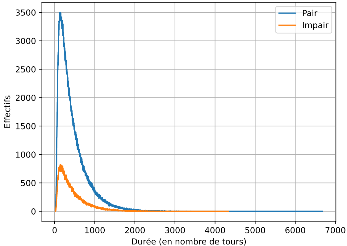
Durées de 1000000 de parties de bataille (4 couleurs de 13 cartes)
