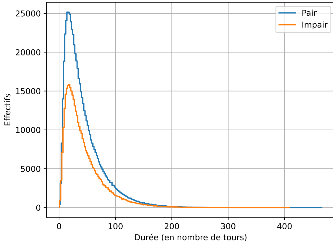
Durées de 1000000 de parties de bataille (7 couleurs de 4 cartes)
