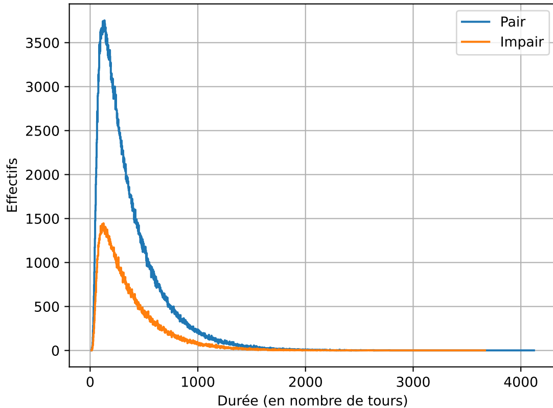
Durées de 1000000 de parties de bataille (7 couleurs de 8 cartes)
